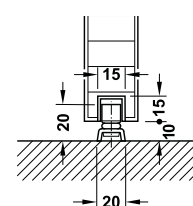
Floor guide with U-shaped guide track in door leaf an floor guide roller Dẫn hướng sàn kèm theo thanh dẫn hướng gắn cửa dạng chữ U và bánh xe
